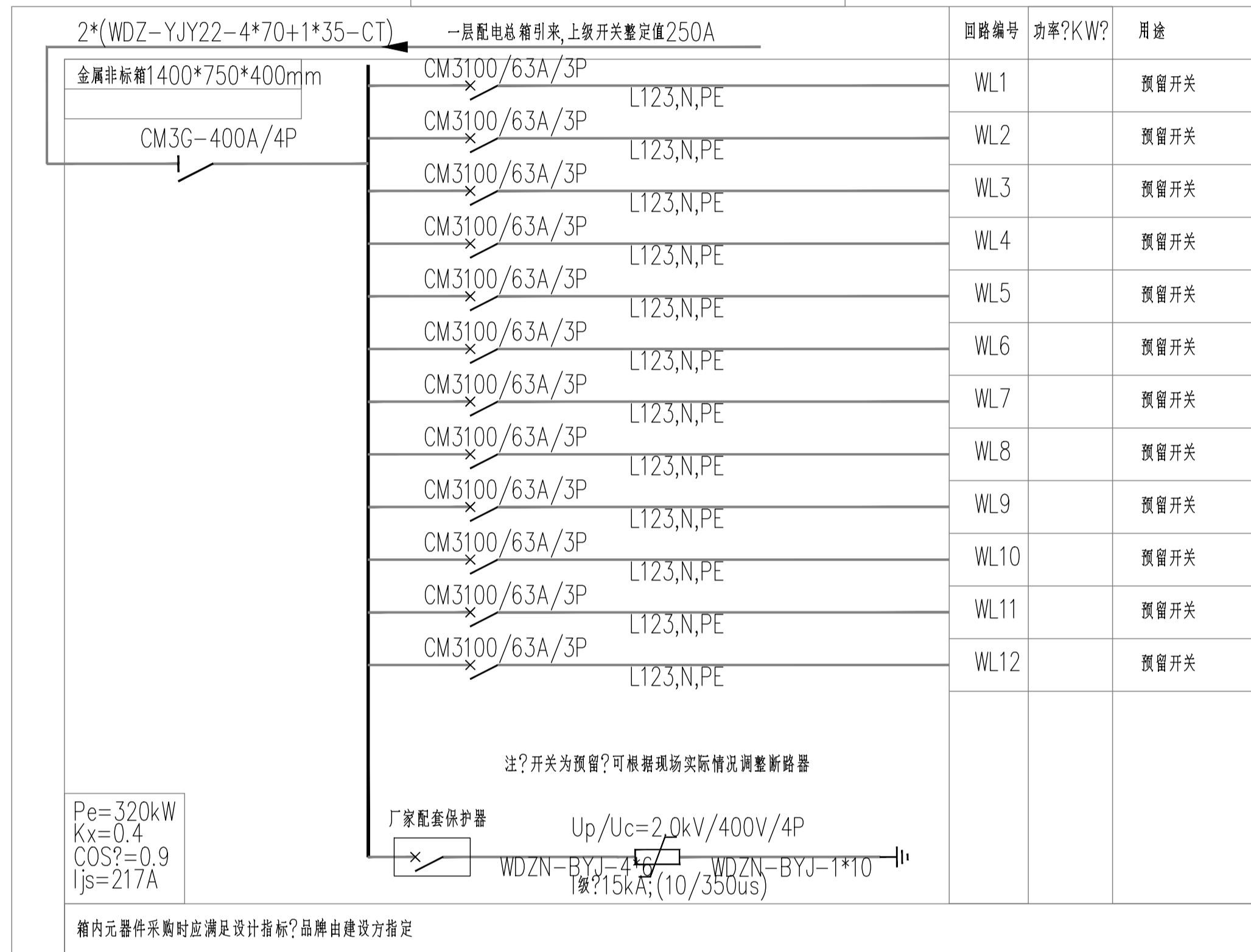
4层新总箱系统图
