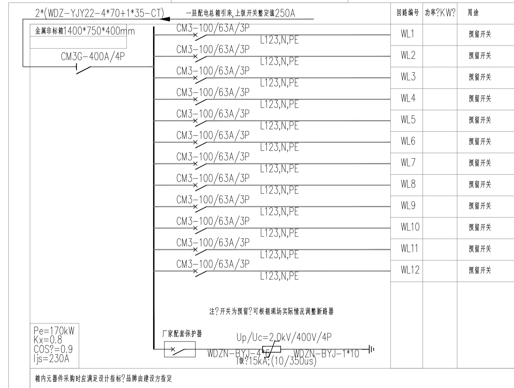
5层新总箱系统图
