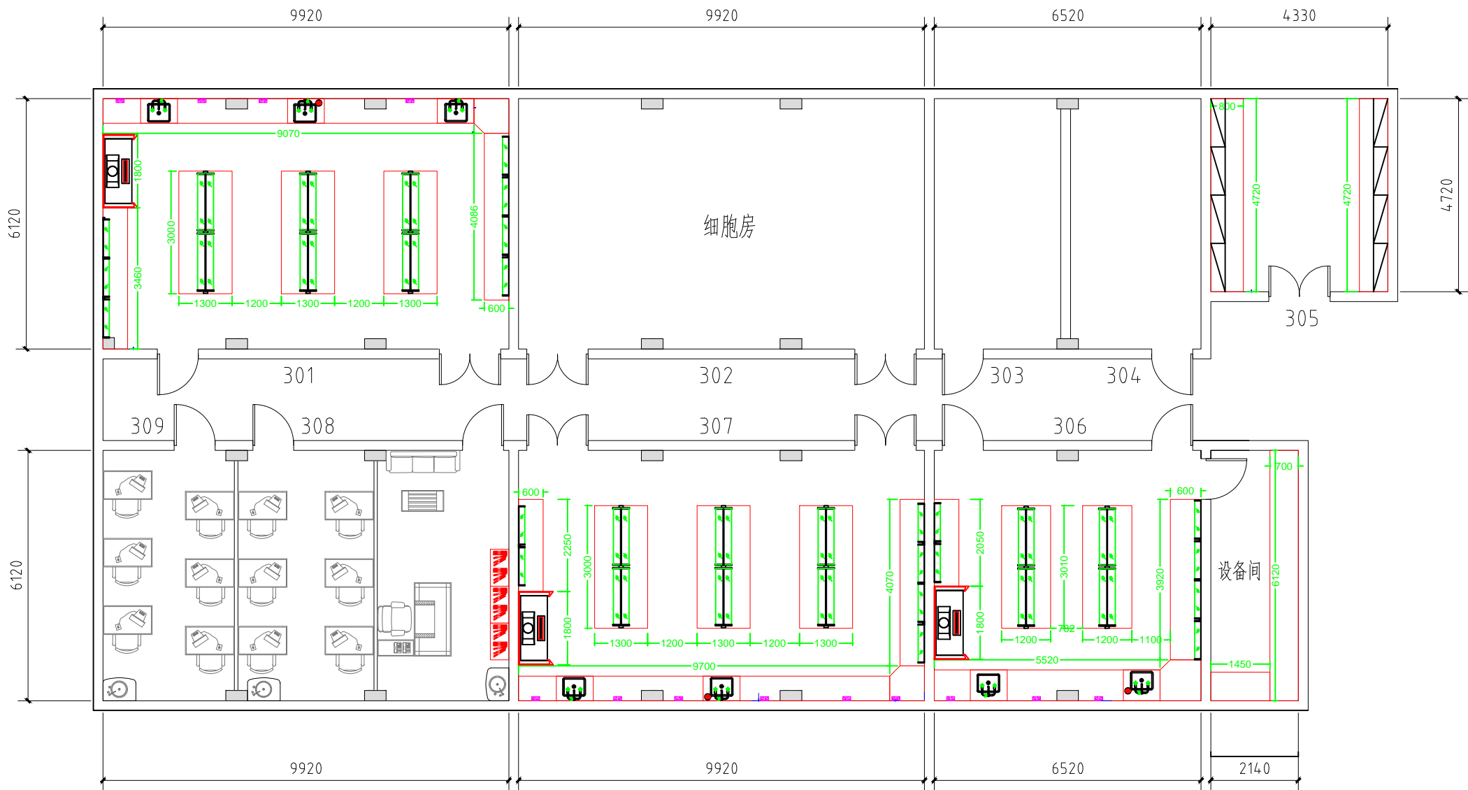
医学院实验室三层平面图
